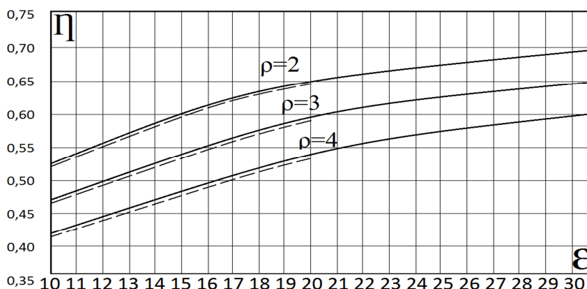
Рис.2 Зависимость термического к.п.д. дизельного двигателя от характеристик \epsilon и \rho
