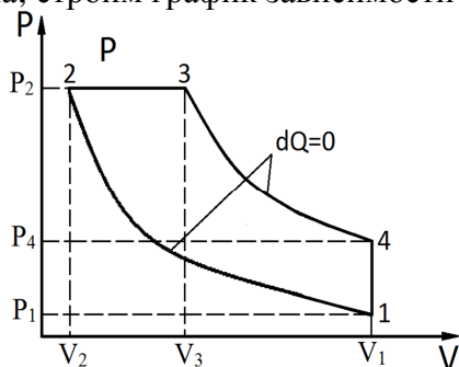
Рис.1 Циклический процесс дизельного двигателя
